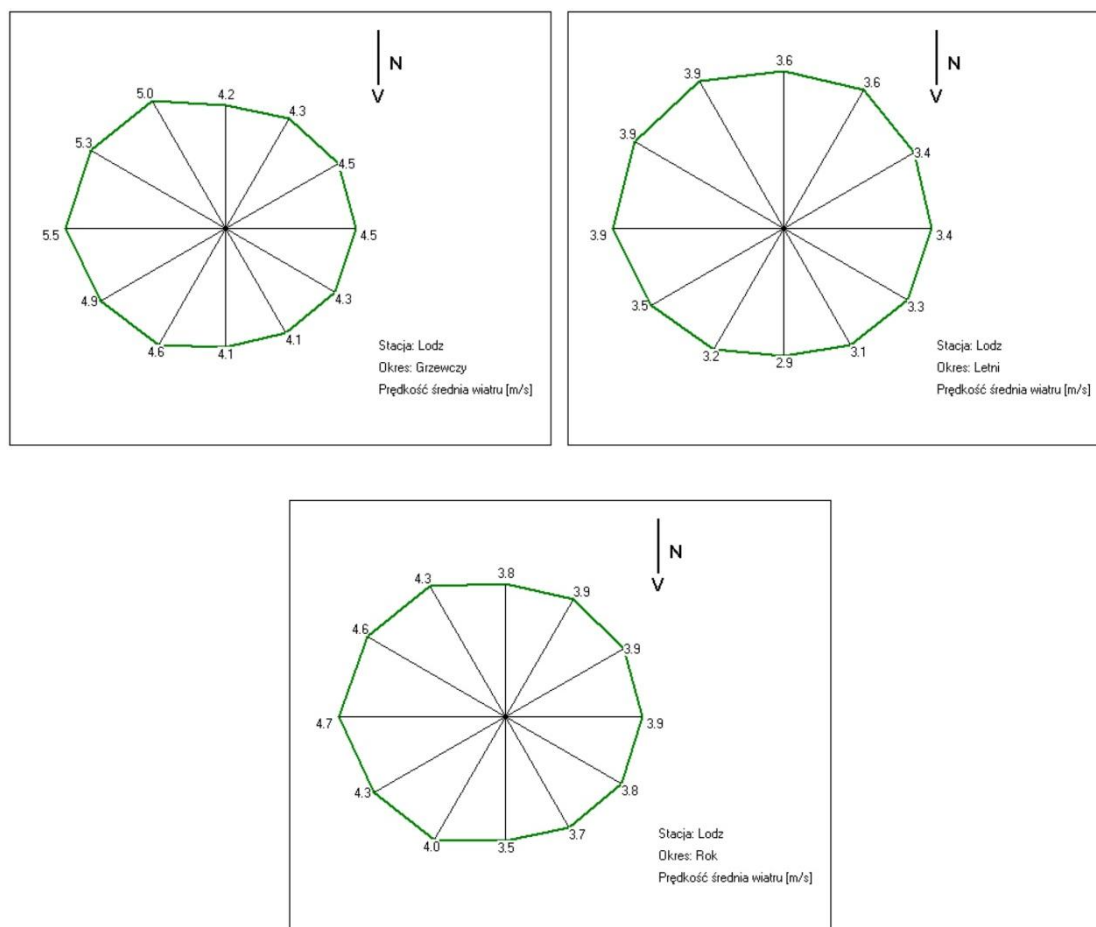
Rysunek nr 16: Prędkość średnia wiatrów dla stacji w Łodzi (róże wiatrów z programu OPA03).
