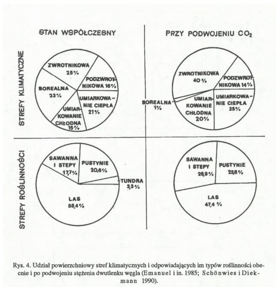
Rysunek 11: Schemat zmian stref klimatycznych i stref roślinności w aspekcie wzrostu stężenia CO w atmosferze.
